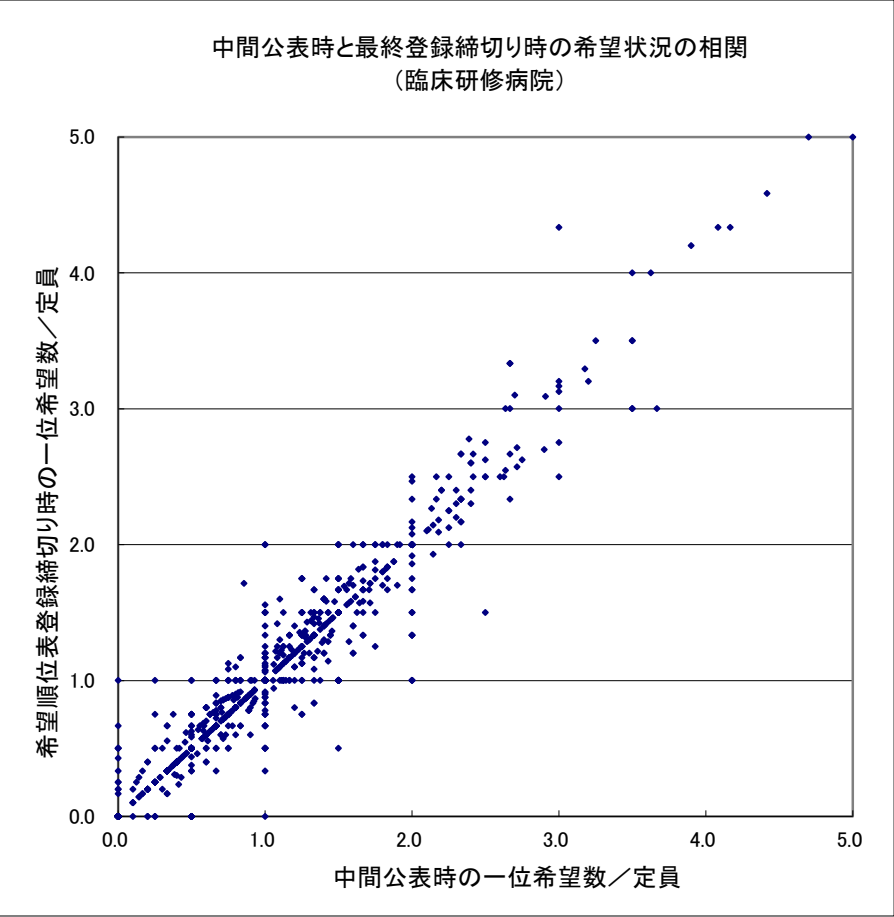
図2. 中間公表時と希望順位表登録締切り時の参加者の一位希望状況の相関 (傾きが1の直線状に分布していれば、中間公表までに希望順位登録を済ませた参加者の数と、最終締切迄に希望順位登録を済ませた者の数が近かったと言える。すなわち、その場合、ほとんどの参加者は中間公表迄に希望順位登録を済ませていたと言える) 中間公表時及び希望順位表登録締切り時のプログラムに対する参加者の一位希望数の相関図を示します。
