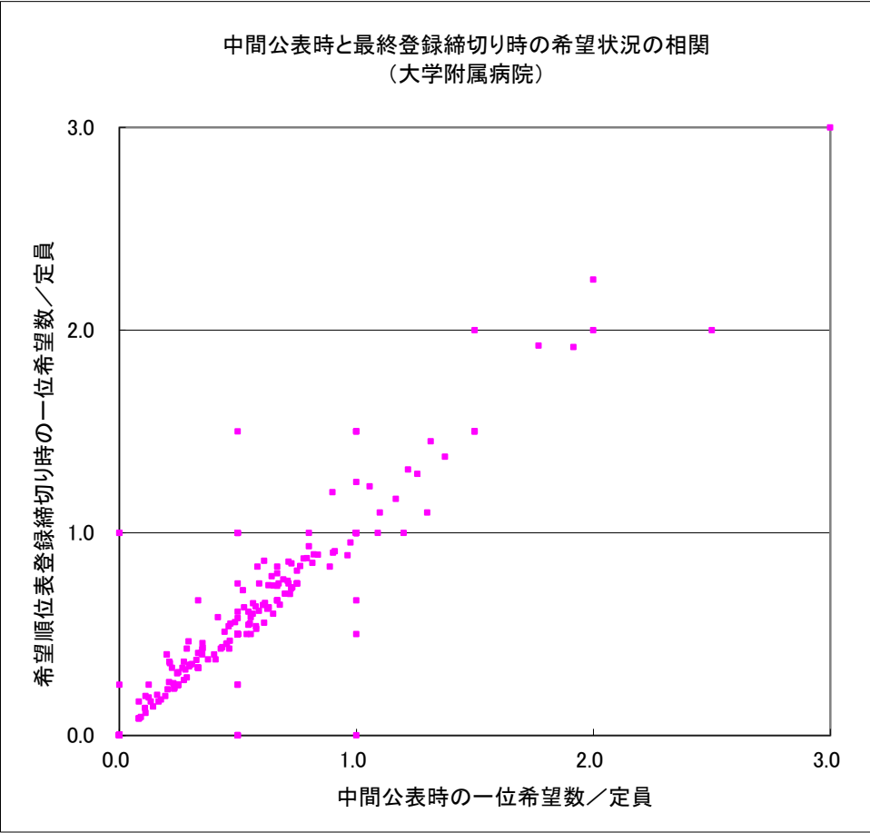
図2. 中間公表時と希望順位表登録締切り時の参加者の一位希望状況の相関 (傾きが1の直線状に分布していれば、中間公表までに希望順位登録を済ませた参加者の数と、最終締切迄に希望順位登録を済ませた者の数が近かったと言える。すなわち、その場合、ほとんどの参加者は中間公表迄に希望順位登録を済ませていたと言える) 中間公表時及び希望順位表登録締切り時のプログラムに対する参加者の一位希望数の相関図を示します。
